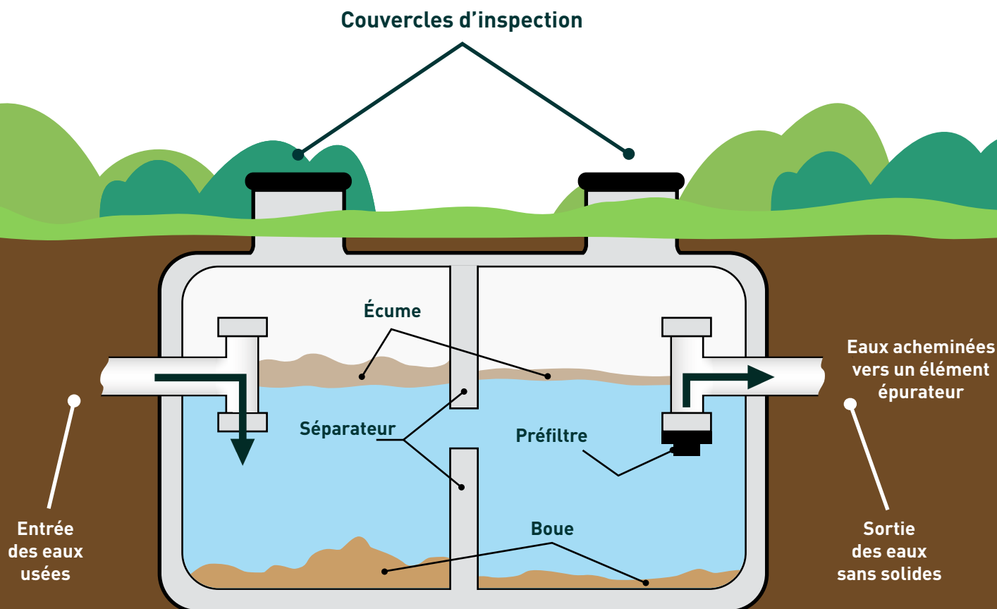
FIGURE 10 : FONCTIONNEMENT D'UNE FOSSE SEPTIQUE
